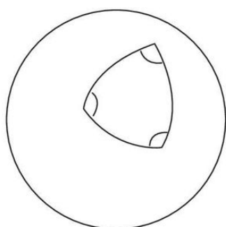
Esfera de radio r , curvatura = \frac{1}{r} > 0
